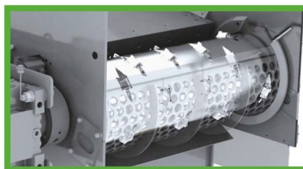
Tamis vissé et échangeable, en plusieurs diamètres d'ouverture pour le tamisage. Extraction par aspiration, possibilité d'extraction par vis ou par bande convoyeuse.
