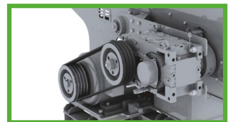
Le rotor est entraîné par un réducteur et une courroie trapézoïdale.
